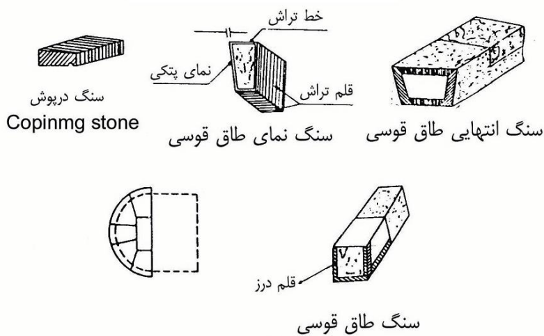
شکل ۲-۵ بنایی با سنگ تمام تراش Moellon Dappareil (FA) Fine Ashlar Masonry
